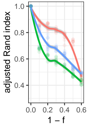
Rand index
