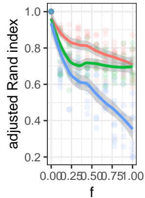
Rand index
