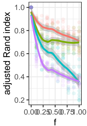
Rand index
