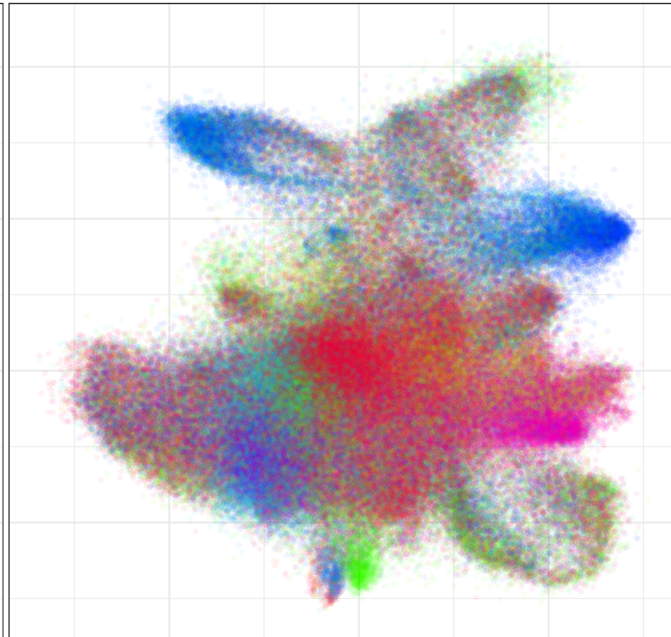
ann
