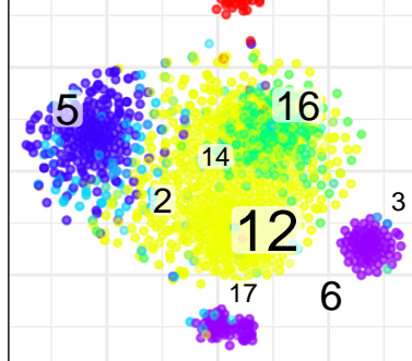
BC2_NORMAL
