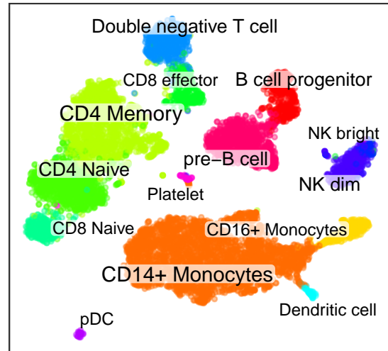
t-SNE
