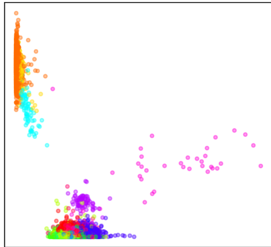
NMF
