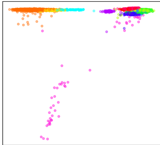
PCA
