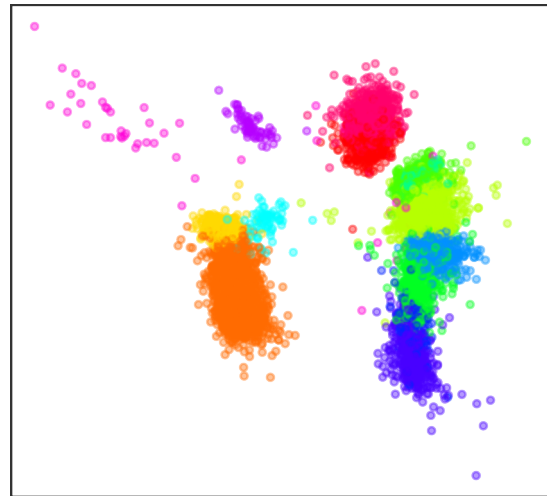
autoencoder
